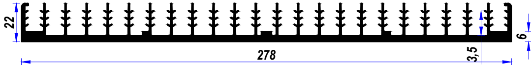
ADS - 278 Alm. Sğt. Prf. Ölçek 1/2
