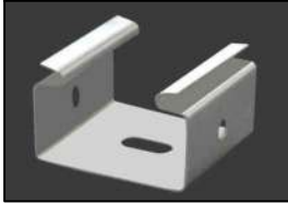
Paslanmaz Klips - H = 12,5mm İçten Kavramalı, sağlam klips
