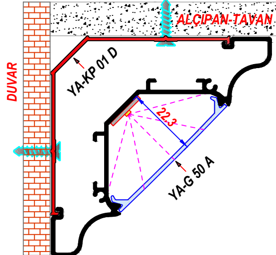
DÜZ DİFÜZÖR
