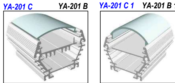
PC.DİFÜZÖR - ALM.PR.F. 610 cm
