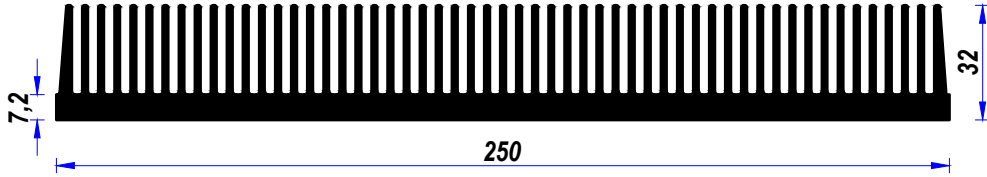
ADS - 250 Alm. Sğt. Prf. Ölçek 1/2
