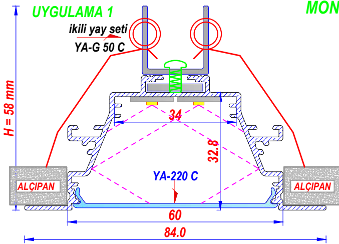
2 FARKLI TAVAN MONTAJ YAYI
