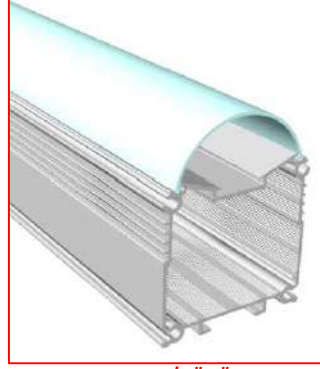
ALM. PRF. - PC. DİFÜZÖR 610 cm
