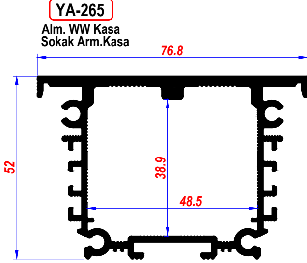
IP 66, SOKAK ARM.-DUVAR BOYAMA KASASI
