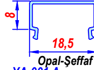
YA-001 A U P.C.Difüzör
