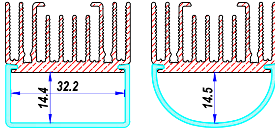
YA-204 C PC. Difüzör YA-204 B
