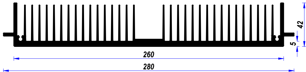
ADS - 280 Alm. Sğt. Prf. Ölçek 1/2
