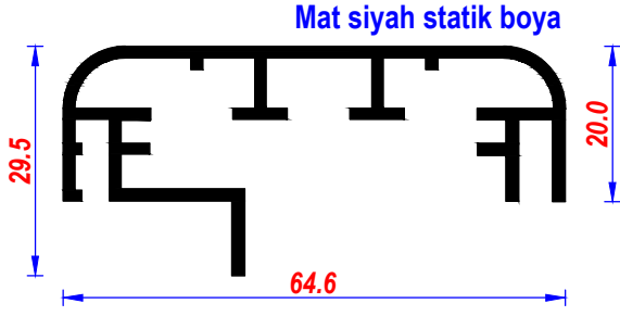
RK - 004 Alm. Kayan Yazı Reklamı Prf.
