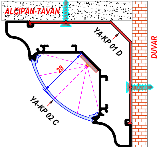
BOMBELİ DİFÜZÖR
