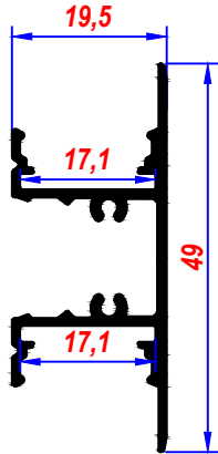
YA - 024 Alm.Led Kasa
