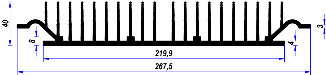
ADS - 267 Alm. Sğt. Prf. Ölçek 1/2
