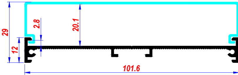
Alm. Reklam Yönlendirme / Led Pef.
