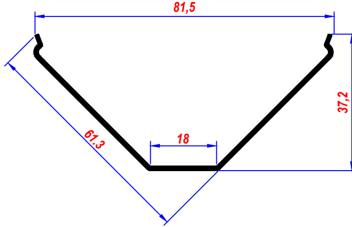
ALM.PRF.-PC DİFÜZÖR 610 cm
