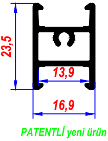
AVZ-017 Alm.Led-Avize Kasa
