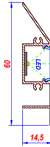
YA-093 Alm. Profil
